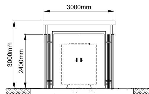
ELEVATION 'D'
